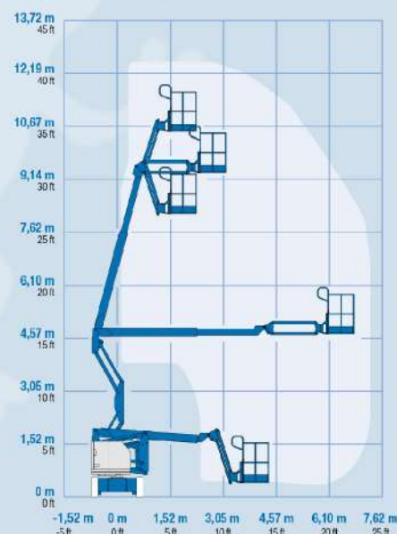
Diagramma di carico Z-34/22N
